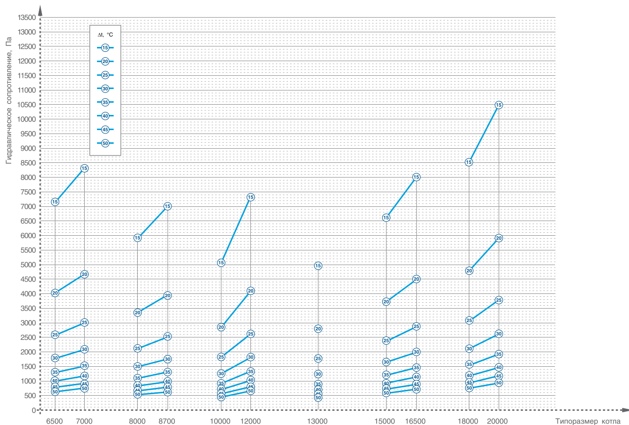
Зависимость гидравлического сопротивления котлов ТТ100-02 от \Delta t . Продолжение
