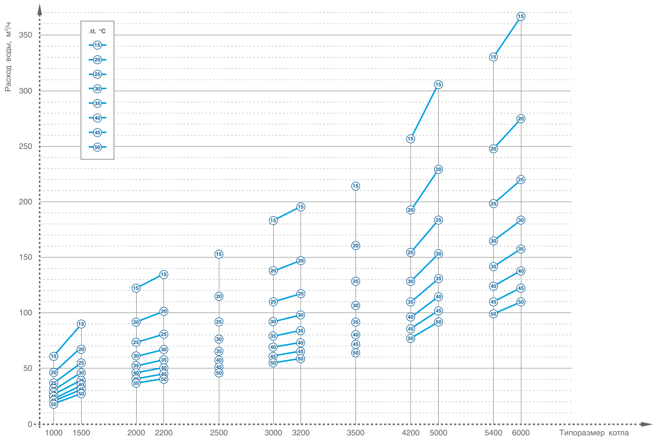
Зависимость расхода воды котлов ТТ100-02 от \Delta t
