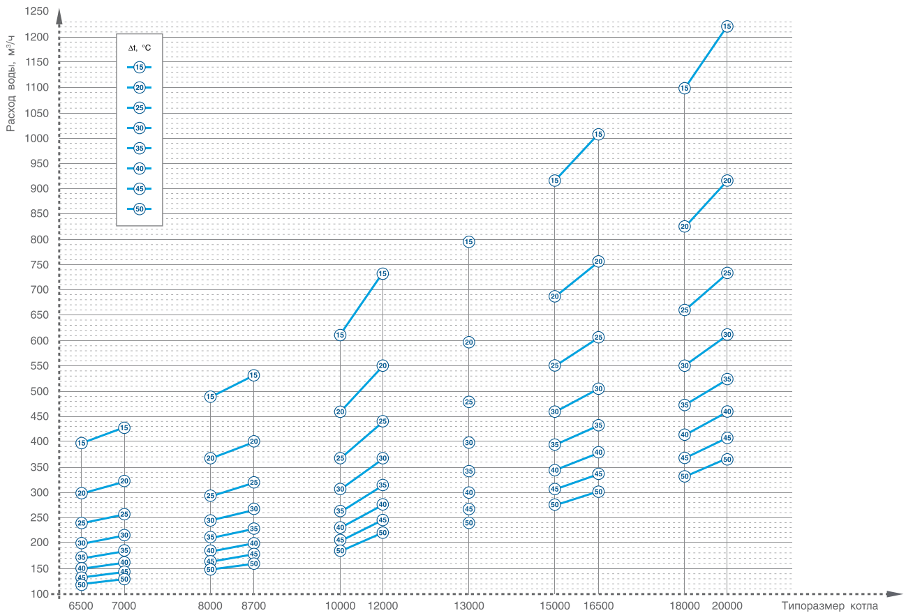
Зависимость расхода воды котлов ТТ100-02 от \Delta t . Продолжение
