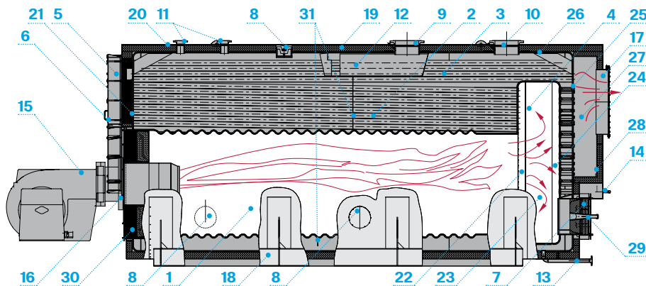
Принципиальная схема работы котла ТТ100-02
