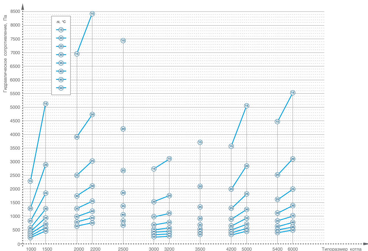
Зависимость гидравлического сопротивления котлов ТТ100-02 от \Delta t
