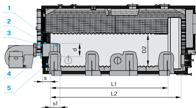
Установка горелки
