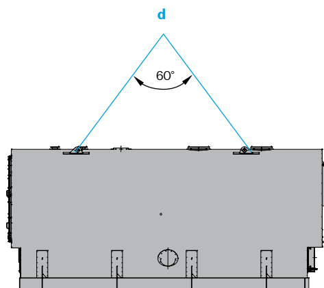
Принципиальная схема строповки котла
