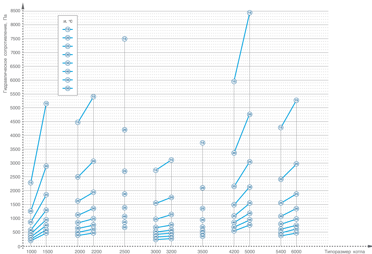
Зависимость гидравлического сопротивления котлов ТТ100 от Δt
