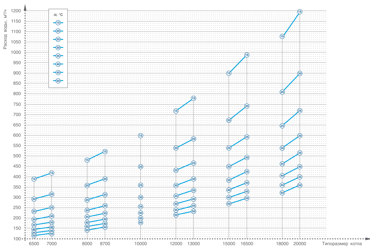
Зависимость расхода воды котлов ТТ100 от \Delta t . Продолжение
