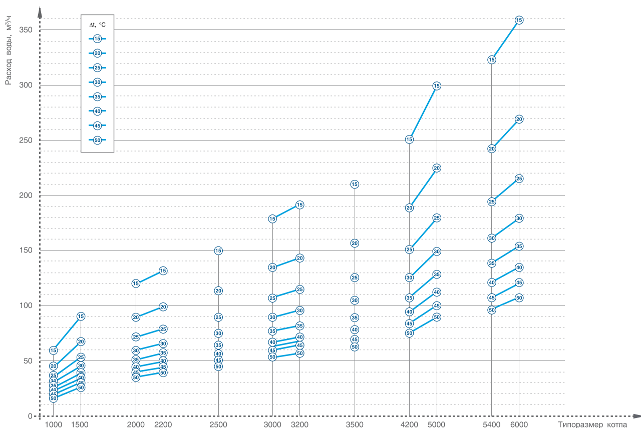
Зависимость расхода воды котлов ТТ100 от \Delta t
