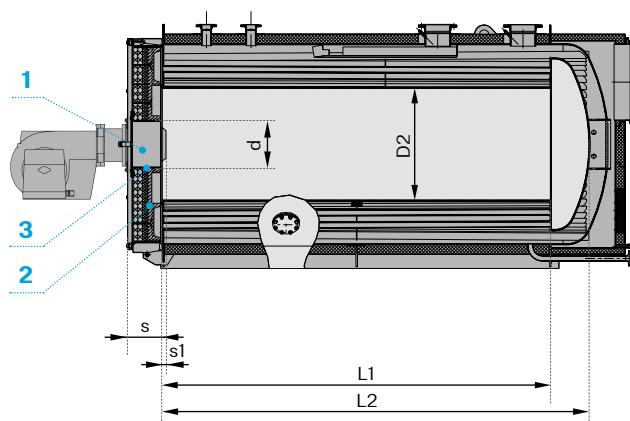
Установка горелки
